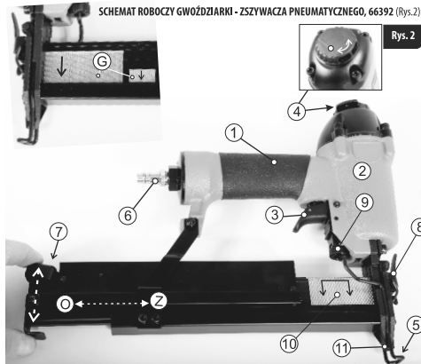
SCHEMAT ROBOCZY GWÓZDIARKI - ZSYWACZA PNEUMATYCZNEGO, 66392 (Rys.2)
