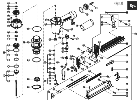
SCHEMAT MONTAŻOWY GWÓZDIARKI - ZSYWACZA PNEUMATYCZNEGO, 66392 (Rys.3)
